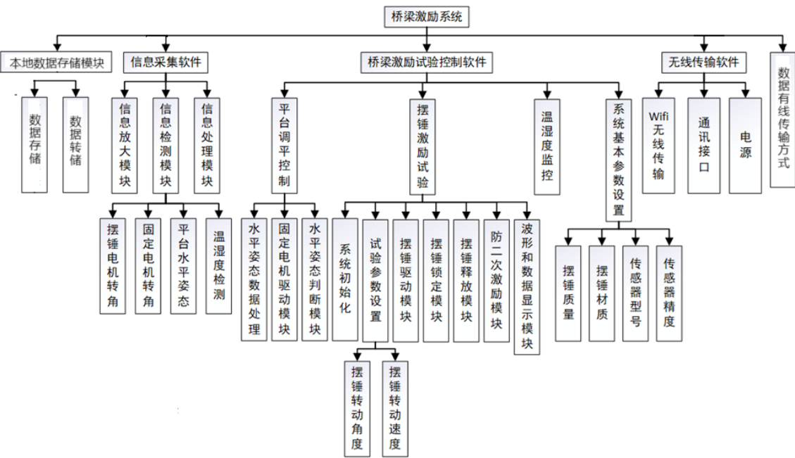
图 3 桥梁自动激励控制系统框图
