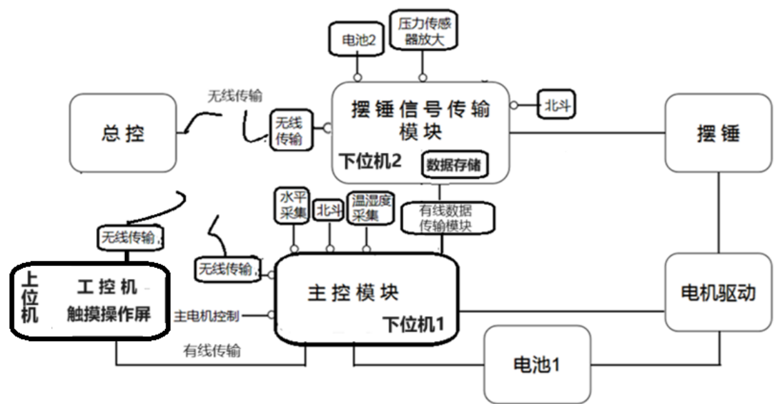
图 1 自动激励控制系统集成设计方案
