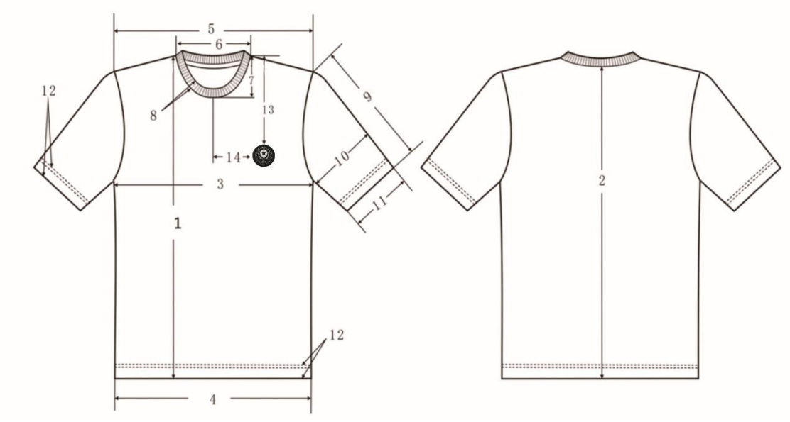
男、女短袖圆领 T 恤衫测量图
