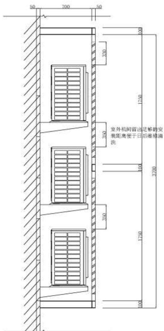
南北两侧空调外机安装示意图
